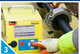
确认管材已刮削和固定
